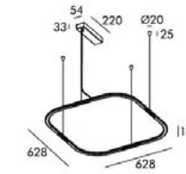
OL 7884 OSRAM SMD
