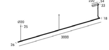
OL 7789 OSRAM SMD
