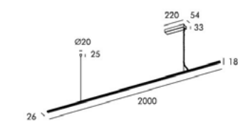
OL 7788 OSRAM SMD
