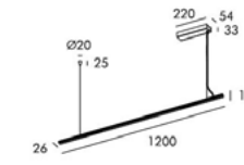
OL 7787 OSRAM SMD
