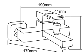
DT-1114 淋浴龙头 Shower mixer 材料 /Material: A 级铜 /Brass
