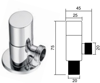
JF-046 角阀 Angle valve 材料 /Material: A 级铜 /Brass
