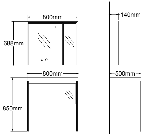
T-9042 LED+Anti-fog 主柜 /Main Cabinet: 800x500mm 镜柜 /Mirror Cabinet : 800x700mm 岩板 /Sintered Stonet : 星空黑 /Sky Black 材质 /Plywood
