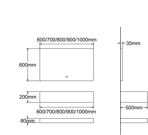
T-10560 台面 /Counter tops: 600x500x200 mm 搁板 /Shelf Borad: 600x500x80 mm 智能镜 /LED Mirror: 500x700 mm 岩板 /Sintered Stone: 意大利浅灰 /Italy Light Grey
