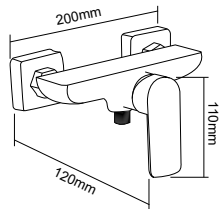
DT-0505 淋浴龙头 Shower mixer 材料 /Material: A 级铜 /Brass
