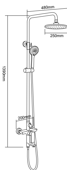
DT-0504 淋浴套件 Shower set 材料 /Material: A 级铜 /Brass
