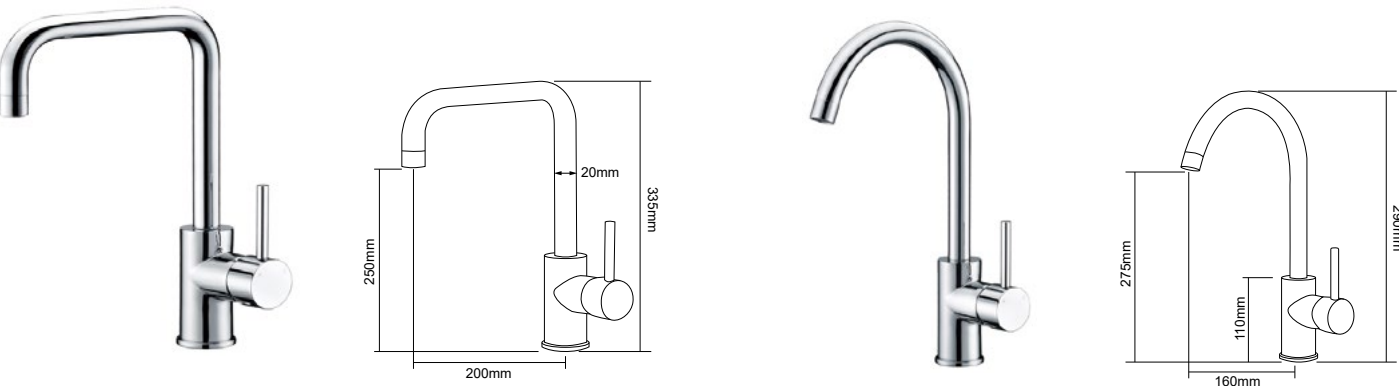
DT-5003 厨房龙头 Kitchen faucet 材料 /Material: A 级铜 /Brass
