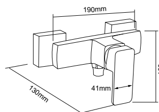
DT-1113 淋浴龙头 Shower mixer 材料 /Material: A 级铜 /Brass
