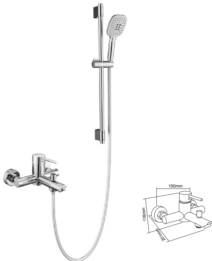
DT-5010 淋浴龙头 Shower mixer 材料 /Material: A 级铜 /Brass
