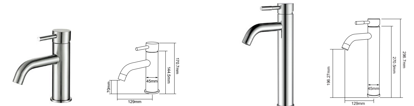
DT-5001 面盆龙头 Basin mixer 材料 /Material: A 级铜 /Brass
