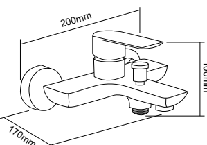
DT-0506 淋浴龙头 Shower mixer 材料 /Material: A 级铜 /Brass
