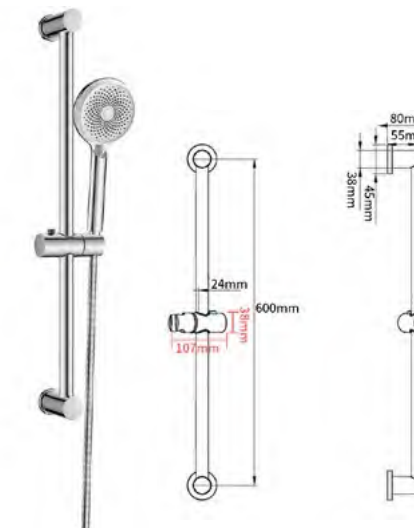
B-23 升降杆 Sliding bar 材料 /Material: 不锈钢 /SUS304
