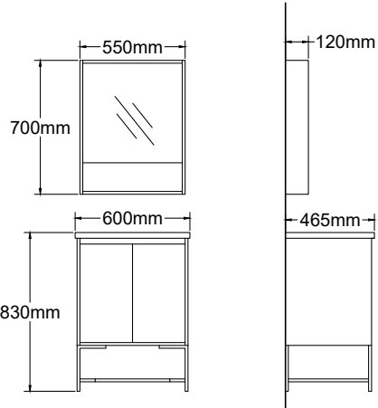
F-5128 主柜 /Main Cabinet: 600x465mm 镜柜 /Mirror Cabinet: 550x700mm 陶瓷盆 /Wash Basin 材质 /Plywood
