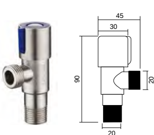
DJF-017BR 角阀 Angle valve 材料 /Material: 不锈钢 /SUS304
