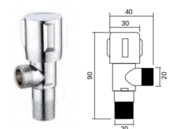
FJF-030 角阀 Angle valve 材料 /Material: A 级铜 /Brass
