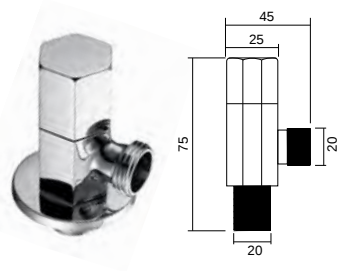
JF-012 角阀 Angle valve 材料 /Material: A 级铜 /Brass
