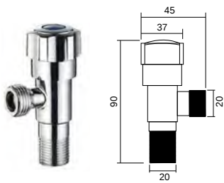
DJF-001 角阀 Angle valve 材料 /Material: 不锈钢 /SUS304
