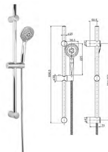
B-24 升降杆 Sliding bar 材料 /Material: 不锈钢 /SUS304
