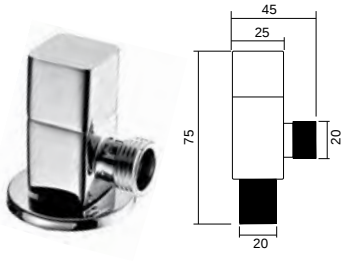
JF-047 角阀 Angle valve 材料 /Material: A 级铜 /Brass
