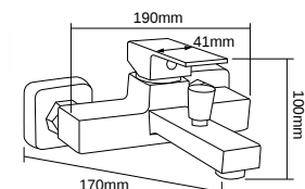
DT-1114 淋浴龙头 Shower mixer 材料 /Material: A 级铜 /Brass
