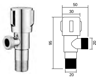
FJF-030BR 角阀 Angle valve 材料 /Material: A 级铜 /Brass
