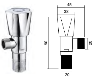
FJF-036 角阀 Angle valve 材料 /Material: A 级铜 /Brass
