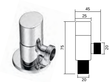
JF-046 角阀 Angle valve 材料 /Material: A 级铜 /Brass
