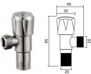
DJF-013 角阀 Angle valve 材料 /Material: 不锈钢 /SUS304
