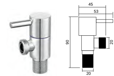
FJF-042 角阀 Angle valve 材料 /Material: A 级铜 /Brass
