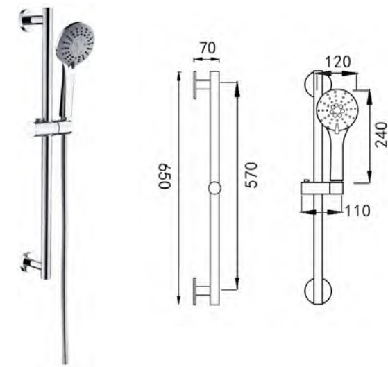
B-15 升降杆 Sliding bar 材料 /Material: 不锈钢 /SUS304
