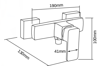
DT-1113 淋浴龙头 Shower mixer 材料 /Material: A 级铜 /Brass
