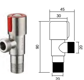
DJF-018BR 角阀 Angle valve 材料 /Material: 不锈钢 /SUS304
