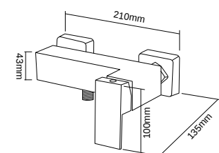
DT-1115 淋浴龙头 Shower mixer 材料 /Material: A 级铜 /Brass
