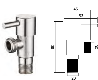
DJF-016BR 角阀 Angle valve 材料 /Material: 不锈钢 /SUS304
