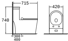
8112 虹吸连体马桶 Siphonic one-piece toilet 尺寸 /Size: 715x420x740 mm 地排 /S-trap, 300/400 mm roughing-in
