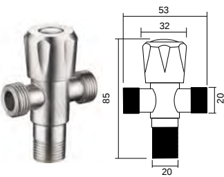
DJF-015BR 角阀 Angle valve 材料 /Material: 不锈钢 /SUS304
