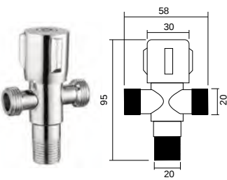
DJF-004 角阀 Angle valve 材料 /Material: 不锈钢 /SUS304
