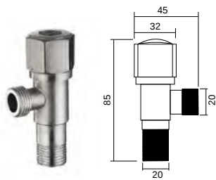
DJF-010BR 角阀 Angle valve 材料 /Material: 不锈钢 /SUS304
